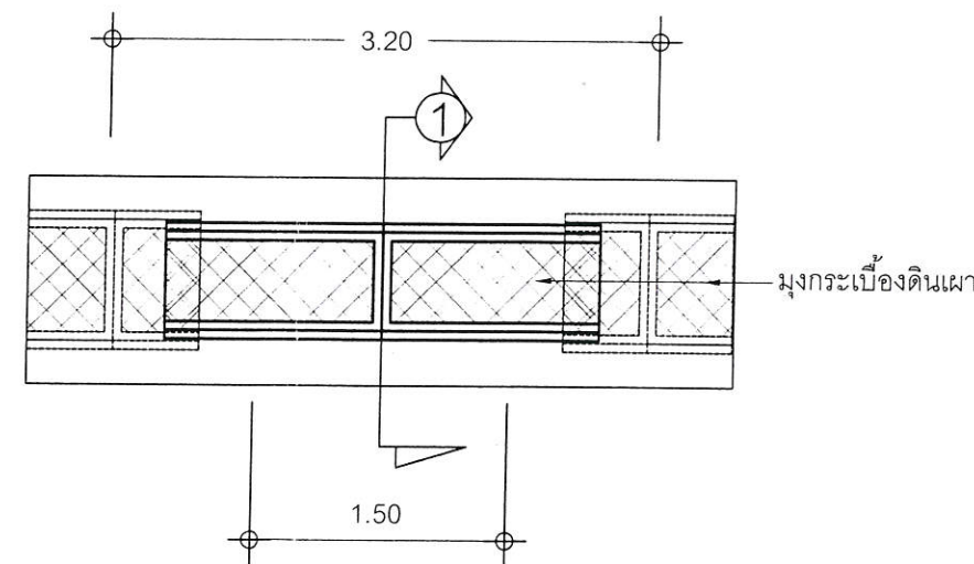
แปลนหลังคา SCALE 1:50
