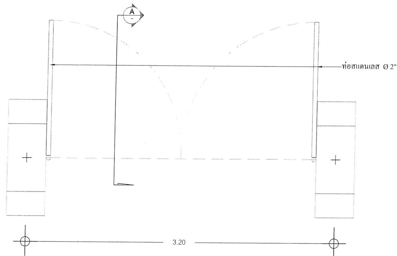
แบบแสดงรายละเอียดประตู NO SCALE
