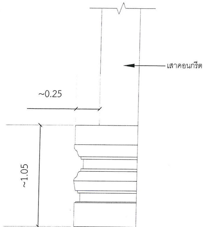
แบบขยายฐานปัทม์ NO SCALE
