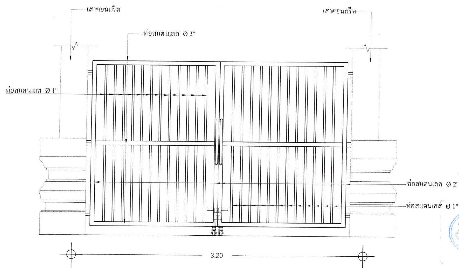
แบบรูปด้านรายละเอียดประตู NO SCALE
