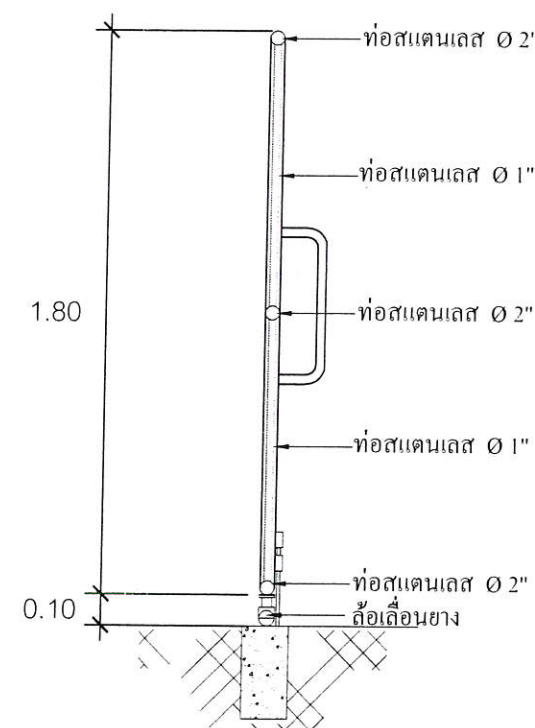
รูปตัดประตู NO SCALE
