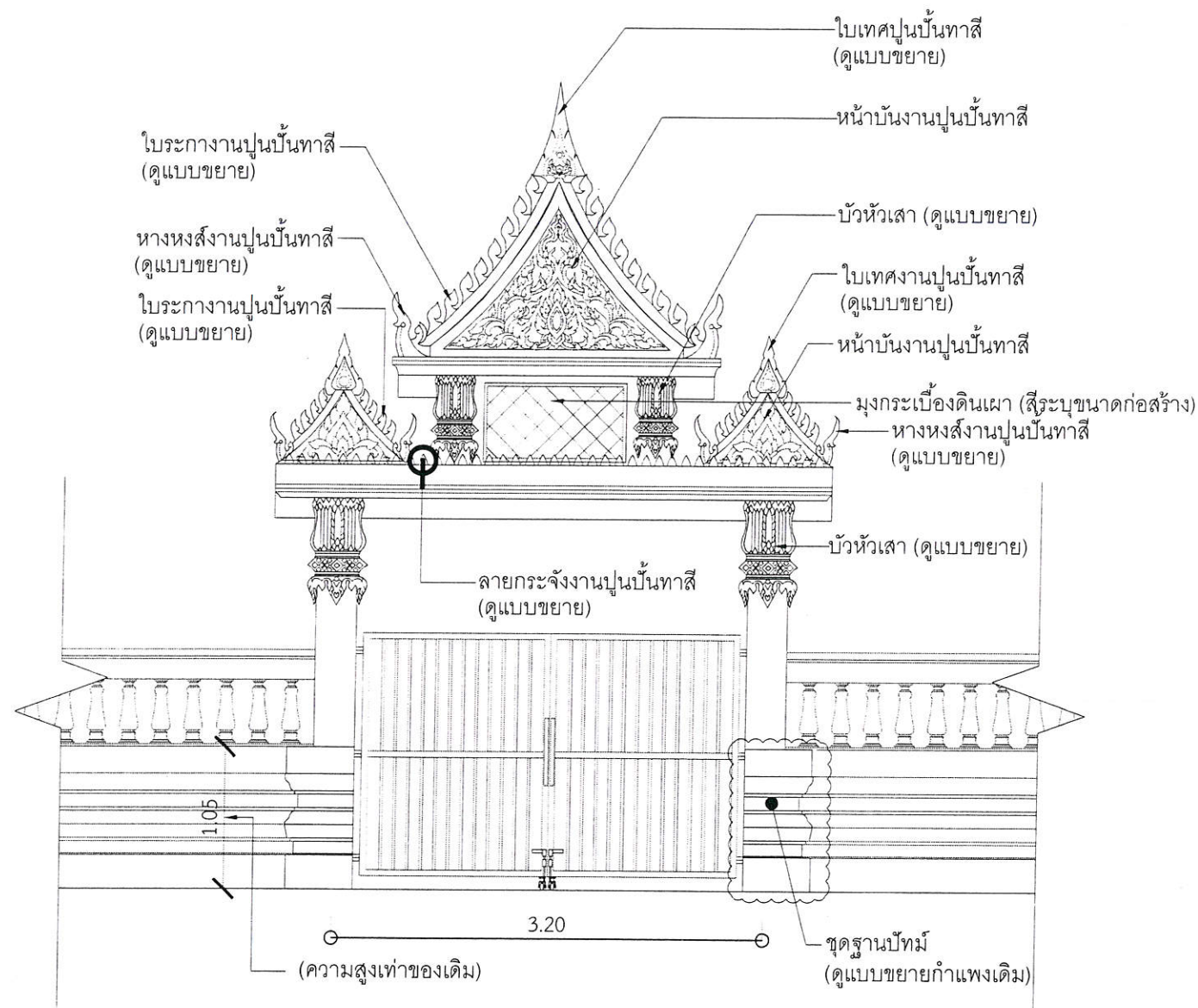
รูปด้านหน้า SCALE 1:50
