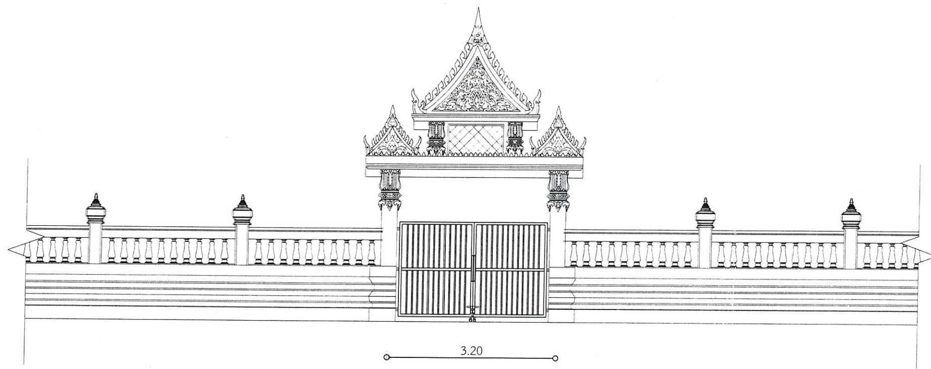
รูปด้านหน้าพร้อมกำแพง SCALE 1:75
