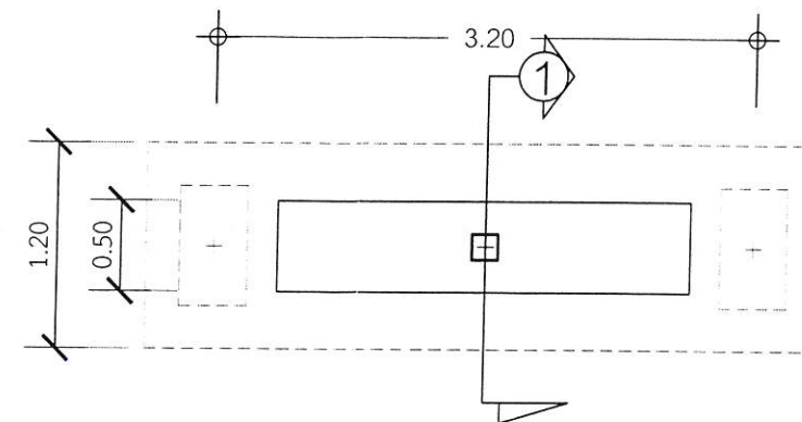
แปลนพื้น ระดับ +3.95 SCALE 1:50
